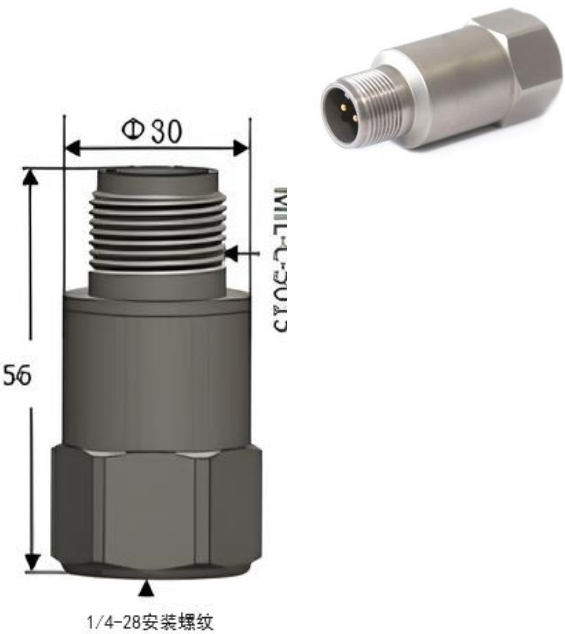
外形示意图
